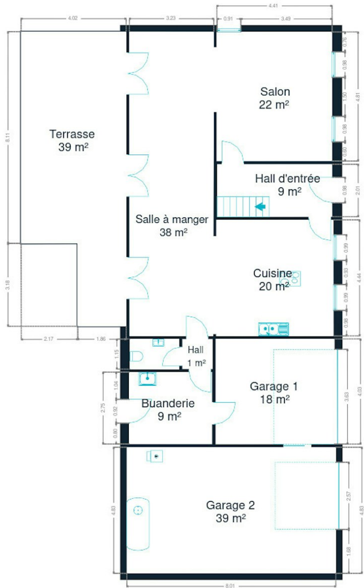
Rez-de-chaussée
